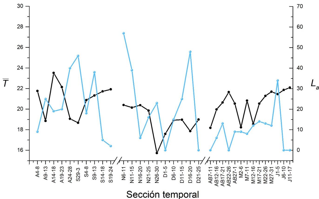
Figura 7. Gráfica que muestra la temperatura promedio \bar{T} (°C) (trazo negro) y la lluvia acumulada L_a (trazo azul) por sección temporal (32 en 7 meses). Los cortes representan las secciones temporales sin datos disponibles. La primera letra de los datos del eje horizontal es la inicial de cada mes y los números son los días del mes abarcados. Para ver a qué mes corresponde cada sección temporal ver anexo 1.
