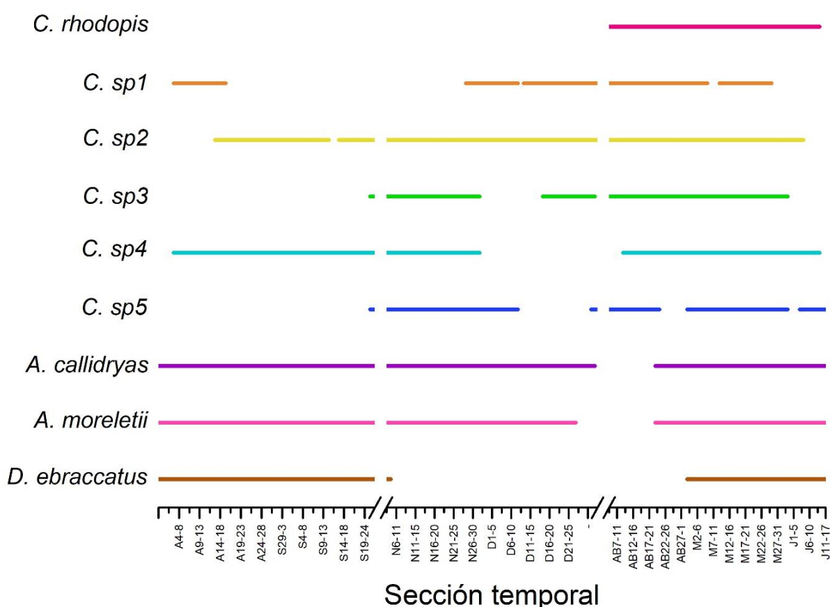
Figura 5. Especies de anuros detectados por el SGA en las secciones temporales registradas (32 en 7 meses), de agosto 2013 a junio 2014 en Nahá, Chiapas. Guiones horizontales indicando la ausencia de registros. La primera letra de los datos del eje horizontal es la inicial de cada mes y los números son los días del mes abarcados. Para ver a qué mes corresponde cada sección temporal ver anexo 1.
